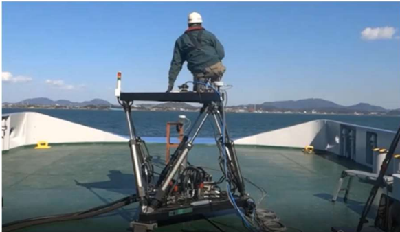
船用動揺吸収装置 揺れないベース
